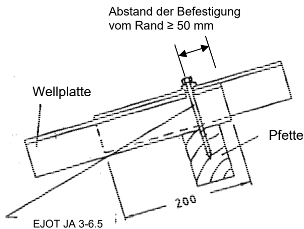
Bild 2.3: Anordnung der Befestigung auf Holzpfetten
