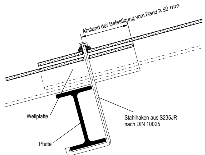
Bild 2.4: Anordnung der Befestigung auf Stahlpfetten
