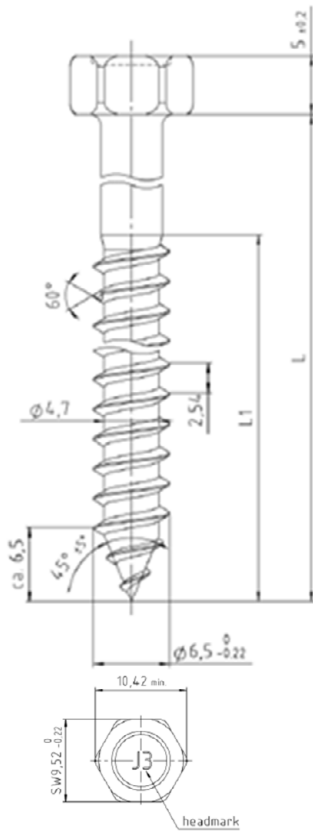
Bild 2.1: Sechskant-Holzschraube EJOT JA3-6,5 x L für Holzpfetten
